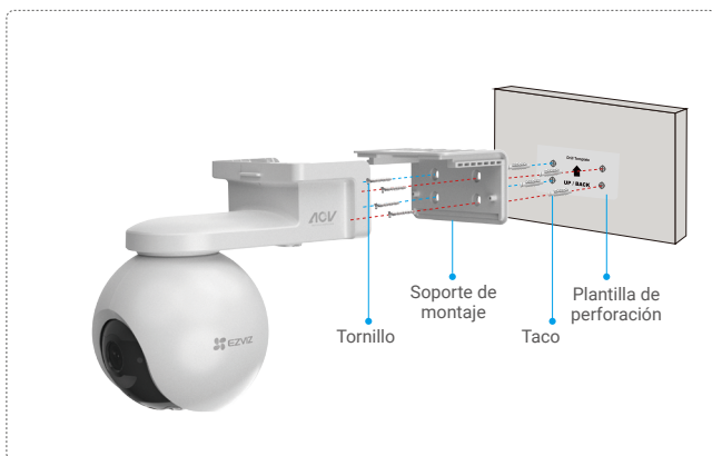
Figura 2. Montaje en pared
