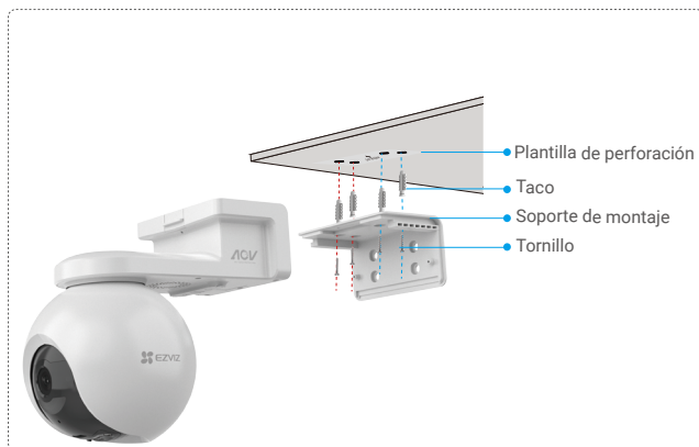
Figura 1. Montaje en techo
